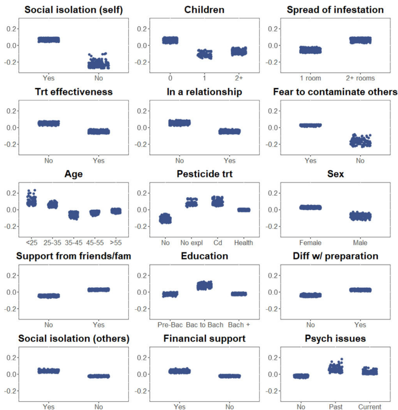
Figure 3. Diagramme de dépendance à une voie SHAPley Additive exPlanations (SHAP) pour les 15 prédicteurs les plus influents. Les valeurs du prédicteur sont représentées sur l'axe x. Les valeurs SHAP sont représentées sur l'axe y. Les valeurs SHAP pour les cinq ensembles de données imputés sont affichées. Une valeur SHAP plus élevée indique une plus grande probabilité de stress élevé lié aux punaises de lit. Légende. Trt, traitement ; fam, famille ; Diff w/, difficultés avec ; Psych, psychiatrique ; No expl, pas d'explication donnée ; Cd, seules les conditions d'utilisation sont expliquées ; Health, problèmes de santé pris en ; Pre-Bac, moins que le baccalauréat ; Bac to Bach, baccalauréat, baccalauréat +1 an, baccalauréat +2 ans ; Bach +, baccalauréat ou plus.
